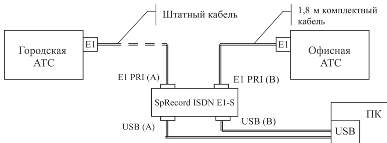
Рисунок 7.1. Подключение адаптера к АТС.
