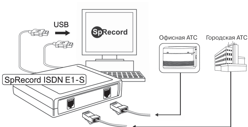
Рисунок 2.1 Система SpRecord.
