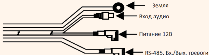
Соединительный кабель
