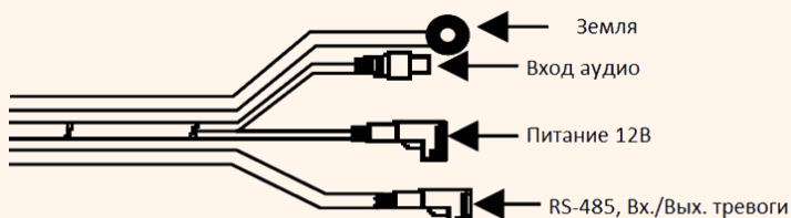
Соединительный кабель
