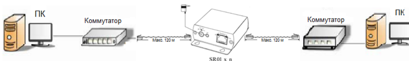
Рис. 6 Схема подключение SR01 к сети Ethernet
